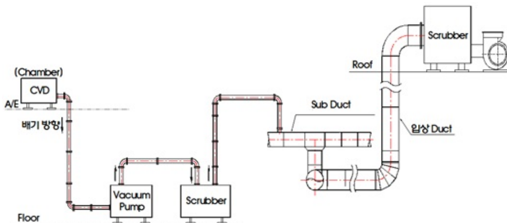
[CVD 공정 이후 혼합배기 흐름도]
